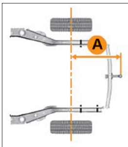
Схема размещения ТСУ (в варианном исполнении)
