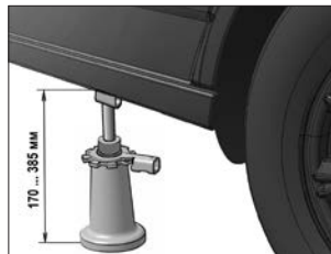
Рис. 3. Положение домкрата при замене колеса
