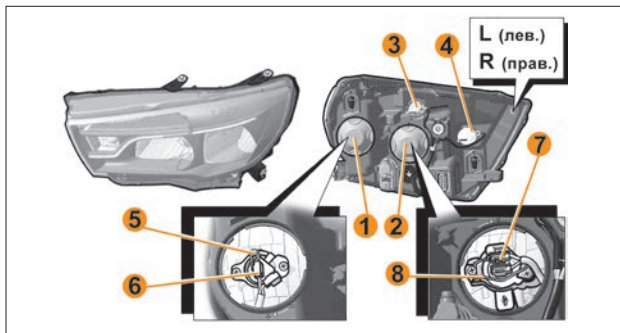
Рис. 11. Блок-фара
