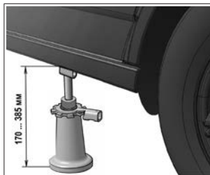
Рис. 3. Положение домкрата при замене колеса
