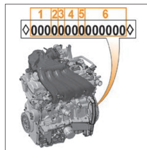
Рис. 2. Маркировка двигателя
