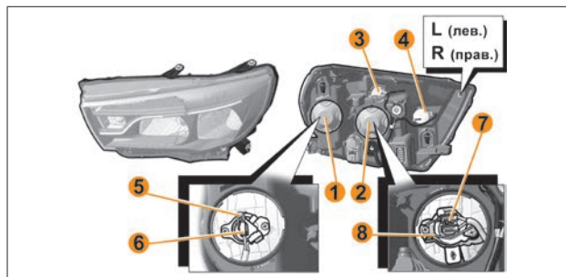
Рис. 11. Блок-фара
