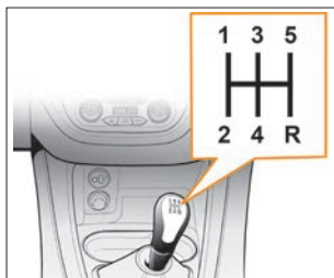
Рис. 19. Рычаг переключения механической коробки передач
