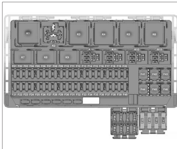
Рис. 3. Расположение предохранителей и реле в монтажном блоке салона
