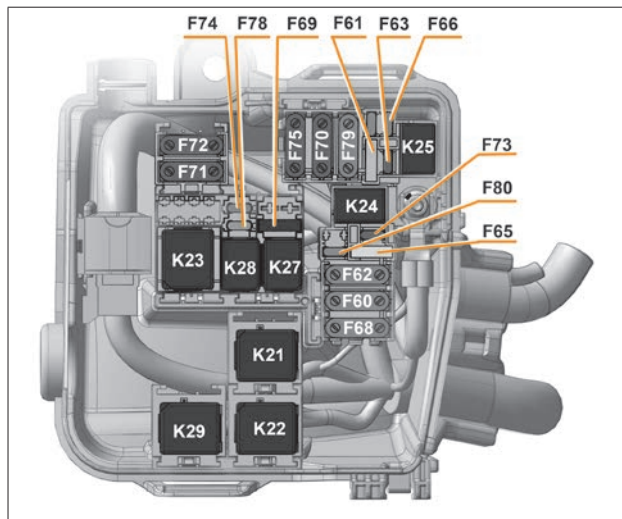
Рис. 1. Расположение предохранителей и реле в монтажном блоке моторного отсека
