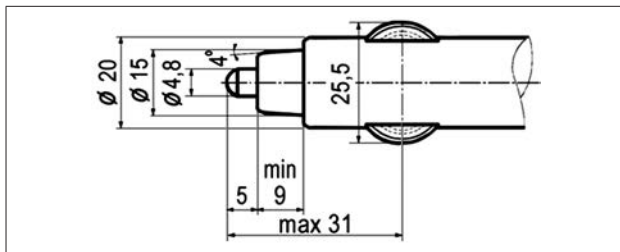
Рис. 3. Вилка электрического прибора для подключения дополнительного электрооборудования
