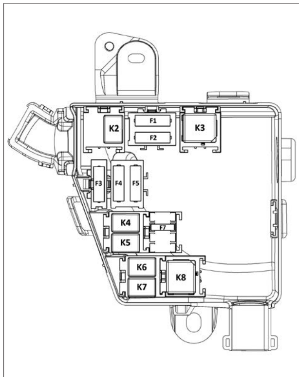
Рис. 3. Блок предохранителей и реле моторного отсека (ДВС K4M)
