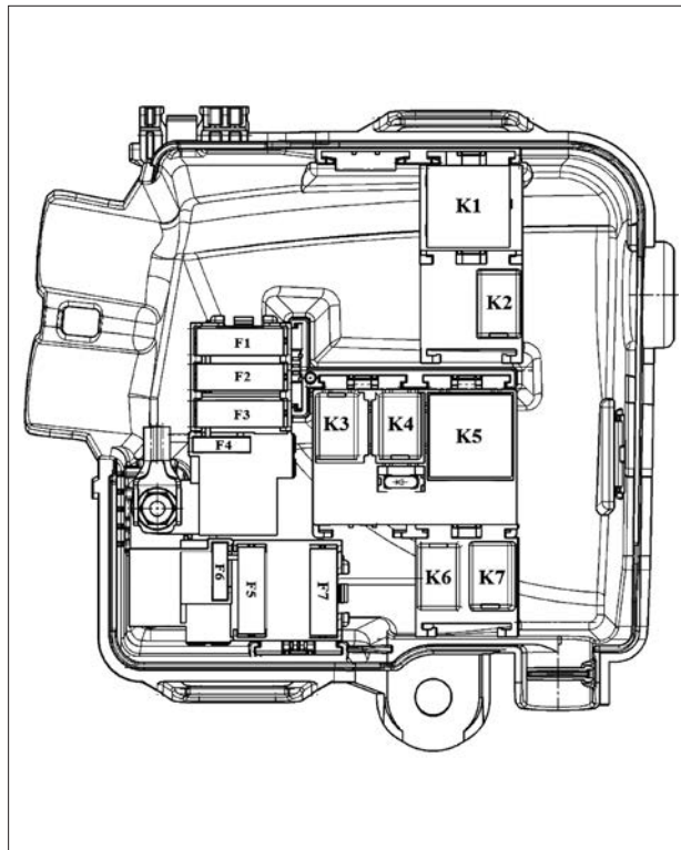
Рис. 2. Блок предохранителей и реле моторного отсека (ДВС 11189)
