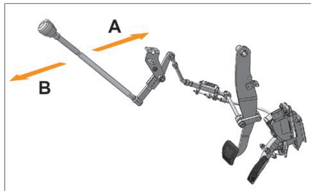
Рис. 3. Устройство ручного управления педалями акселератора и тормоза для автомобилей с автоматизированной (АМТ) коробкой передач и левым расположением органов управления
