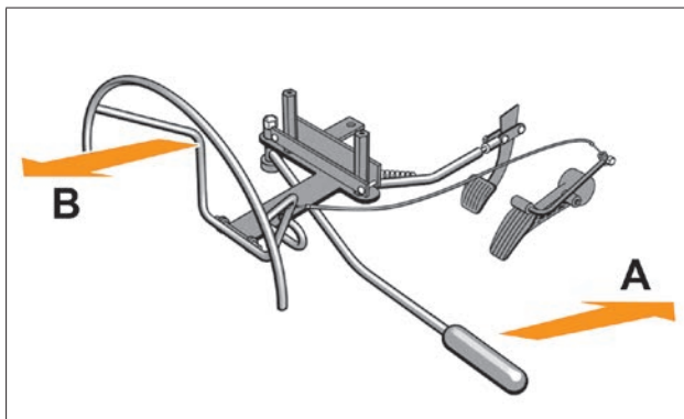
Рис. 2. Устройство ручного управления педалями акселератора и тормоза для автомобилей с автоматизированной (АМТ) коробкой передач и правым расположением органов управления
