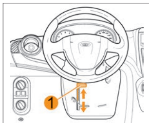
Рис. 12. Регулировка положения рулевого колеса (в варианном исполнении)
