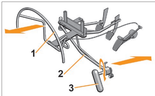
Рис. 4. Устройство ручного управления педалями акселератора, тормоза и сцепления для автомобилей с механической коробкой передач (МКП) и правым расположением органов управления
