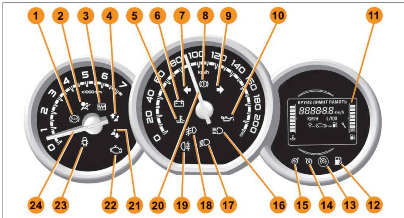
Рис. 3.2.1. Комбинация приборов (в варианном исполнении)
