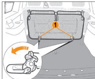
Рис. 2.3.5. Защелки крепления сиденья третьего ряда
