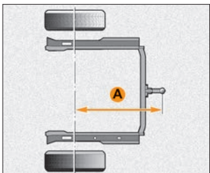
Рис. 5.15.1. Схема размещения ТСУ (в варианном исполнении)
